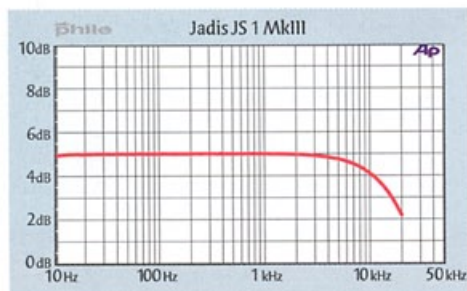
Abb. 1: Zugunsten besserer Impulswiedergabe fallen die Höhen prinzipbedingt etwas ab.
