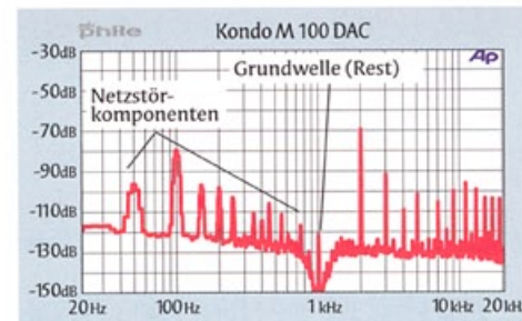
Abb. 4: Im Klirrspektrum dominiert die erste Oberwelle ( k_2 ); der Netzbrumm stört kaum.
